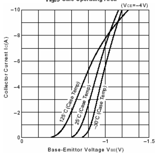
Fig.7 I_C-V_{BE}
