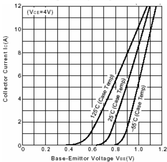
Fig.7 I_c - V_{BE}
